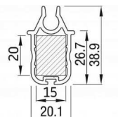
End Slat
